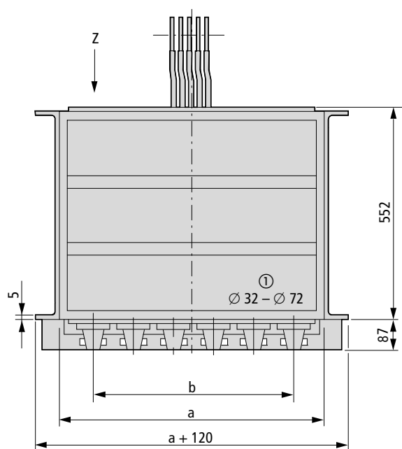
Вид спереди
