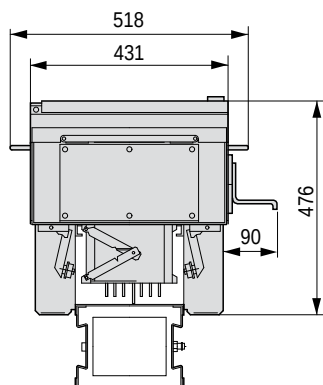
Отводной блок с дверцей
