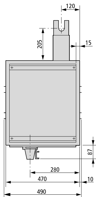
Вид сбоку
