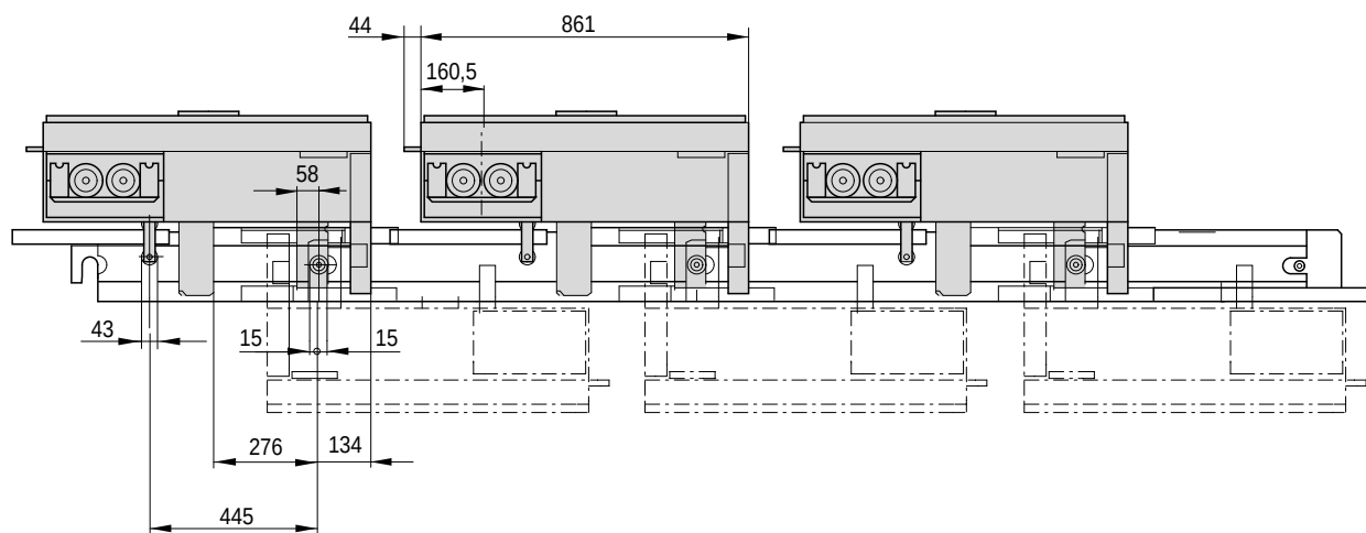
Отводной блок с дверцей
