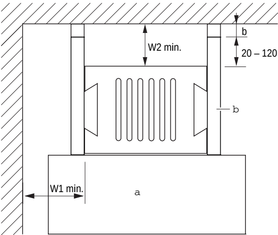
a Отводной блок a LD-BV Вертикальный кронштейн подвеса
